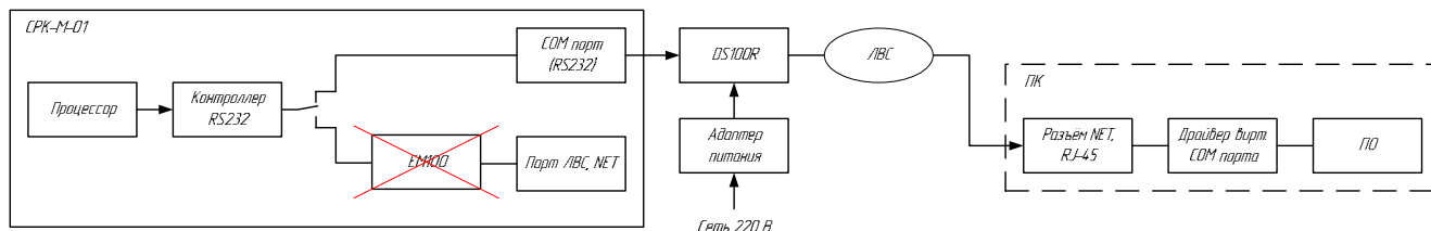
Рисунок 3 – Подключение через внешний модуль RS232-Ethernet
