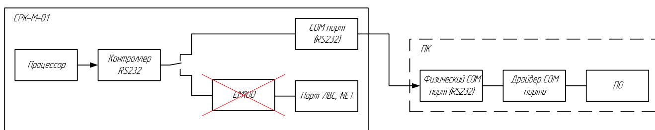
Рисунок 1 – Схема прямого подключения по RS232
